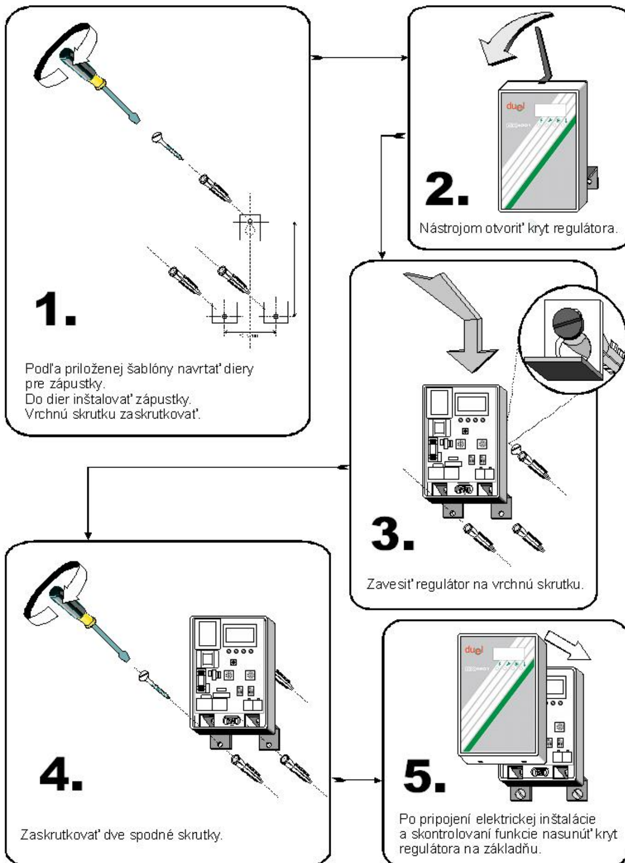
Obr.13 Montáž prístroja
