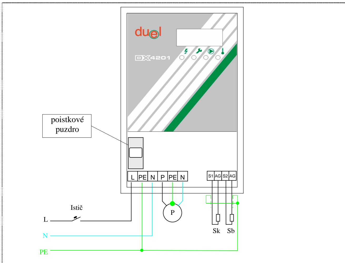
Obr.14 Príklad zapojenia regulátora DX4201 (svorkovnica a poistkové puzdro sú pod krytom): Sk - snímač teploty kolektora, Sb - snímač teploty výmenníka, P - čerpadlo
